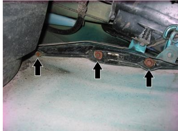
6. Nu ser du de 3 skruvarna som håller stötfångaren mot framskärmen (bild tagen underifrån), lossa dessa (den bakre sitter skruvad uppifrån)
